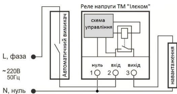
Схема 1. Монтажна схема реле напруги РН-32/40/63
